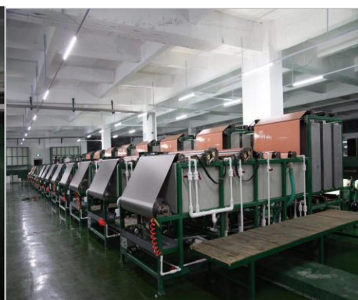
材料涂胶成半成品
